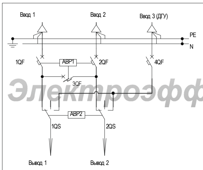
Схема 420 - 3 ввода (2 ввода от сети + 1 ввод от ДГУ), 2 вывода, 1 секц. аппарат
